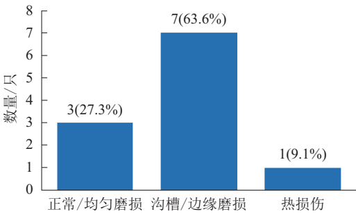
图1 典型出孔钻头主导形态统计
