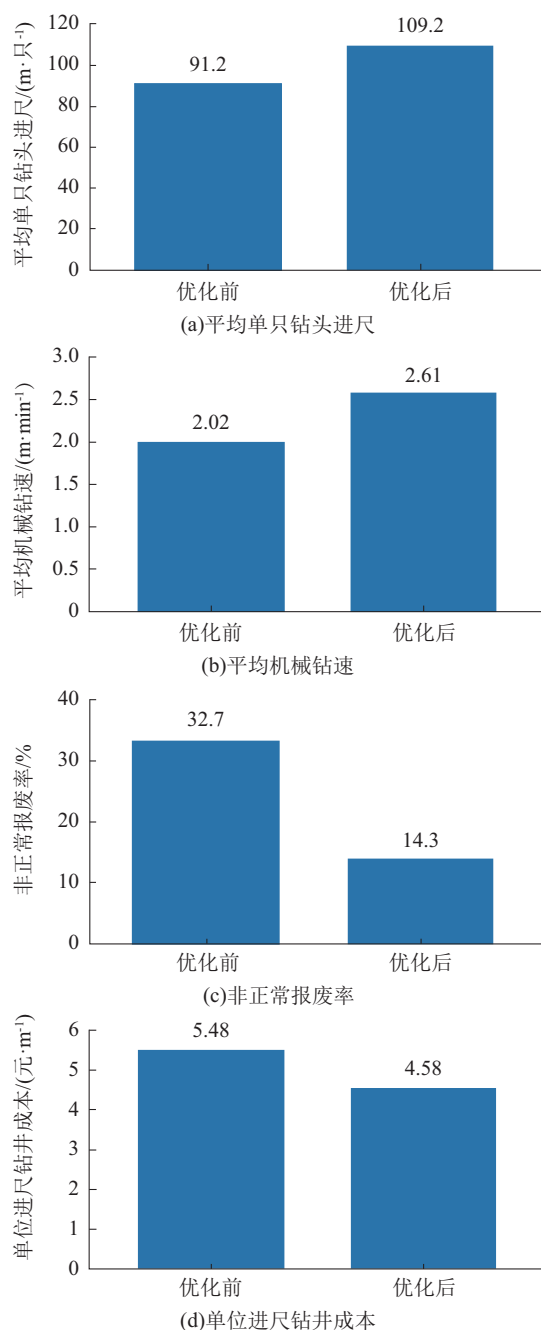
图3 优化前后主要指标对比
