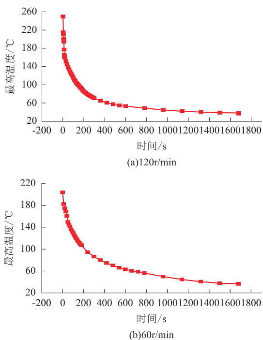
图8 不同转速下PDC钻头降温曲线
