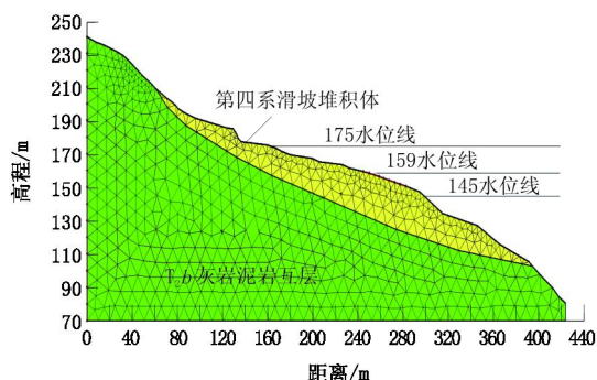
图2 计算模型
