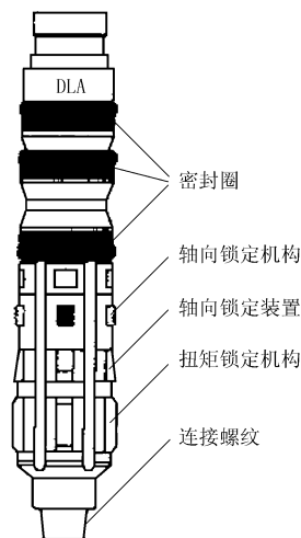
图 2 锁定机构总成
