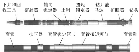
图 1 TESCO 公司的一种井下回收工具
