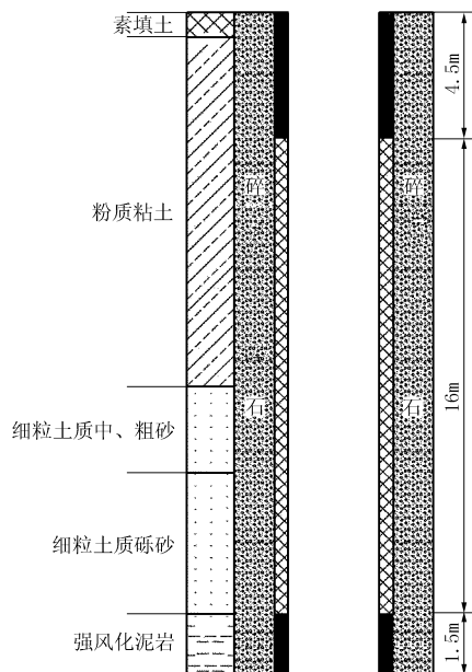
图1 主井成井示意图
