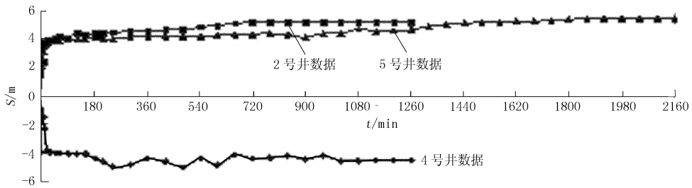
图 2 抽水试验的 S-t 曲线图
