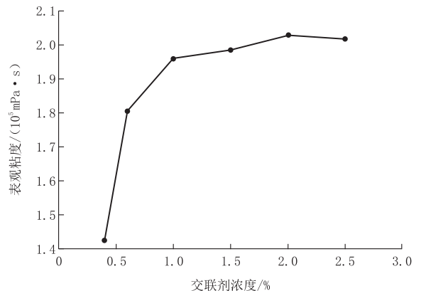
图 2 交联剂浓度对表观粘度的影响
