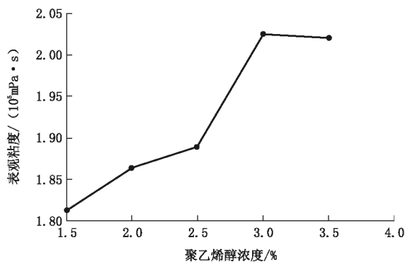
图 1 聚乙烯醇浓度对表观粘度的影响
