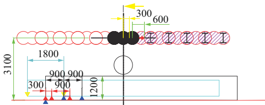
图 6 桩位对中
