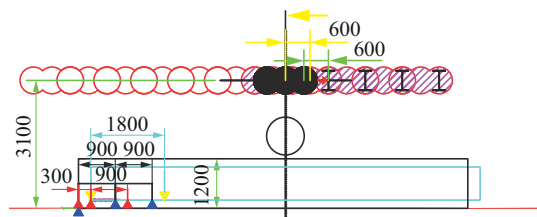
图 4 插放第 1 根型钢
