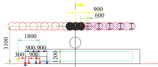
图 5 插放第 2 根型钢
