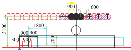
图 3 施工套打幅
