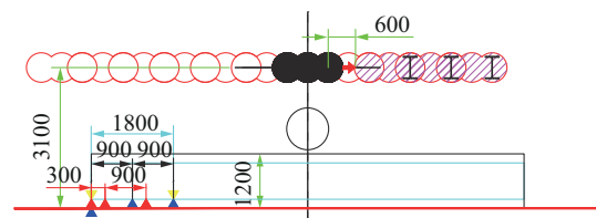
图2 施工跳打幅
