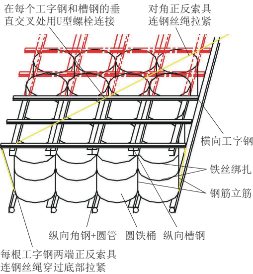
图3 水上钻探平台桶排框架局部结构示意图 Fig.3 Local structure of the barrel frame of the waterborne drilling platform
