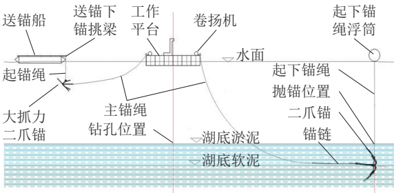
图4 一种用于深水湖泊水上钻探工作平台锚固定位的大抓力二爪锚装置
