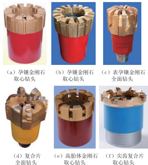
图6 工程应用中的金刚石钻头 Fig.6 Diamond bits for engineering application
