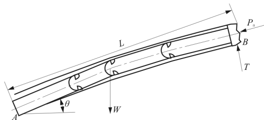
图1 挠性钻具受力示意图
