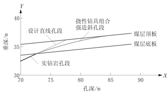
图5 1-3号孔轨迹图
