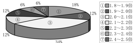
图6 20个20°~40°倾角的钻孔煤孔段延伸率统计图
