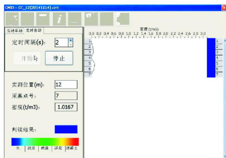
图5 定时自动采集
