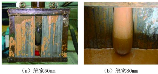
图5 堵漏袋在模拟垂直裂缝中封堵情况
