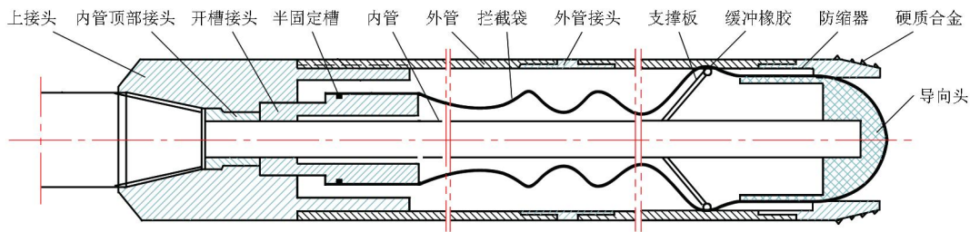
图 1 拦截式堵漏工具结构
