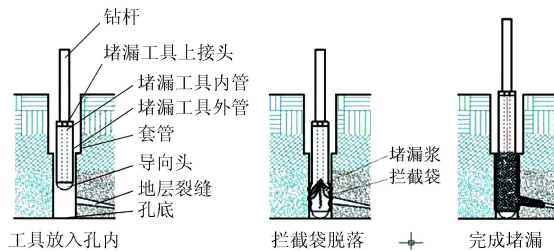
图 3 拦截式堵漏工具堵漏示意图
