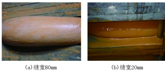
图6 堵漏袋在模拟水平裂缝中封堵情况
