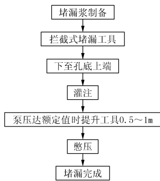
图 2 拦截式堵漏工艺流程图
