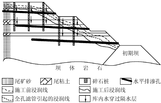
图 1 尾矿库联合排渗示意图
