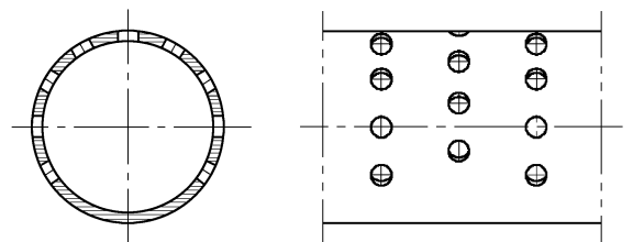
图 2 “导水滤管”示意图
