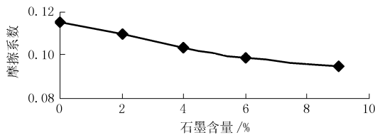
图4 摩擦系数与石墨含量的关系
