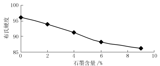
图 2 石墨含量对胎体硬度的影响
