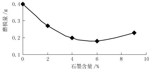
图3 磨损量与石墨含量的关系
