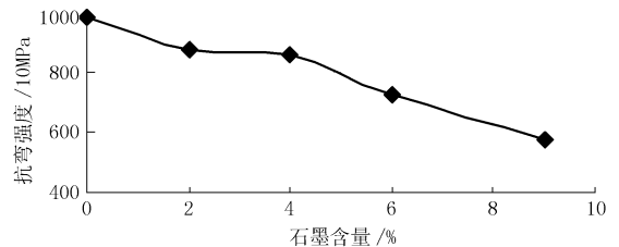
图 1 石墨含量对抗弯强度的影响
