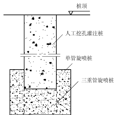
图 2 旋喷桩加固处理剖面图
