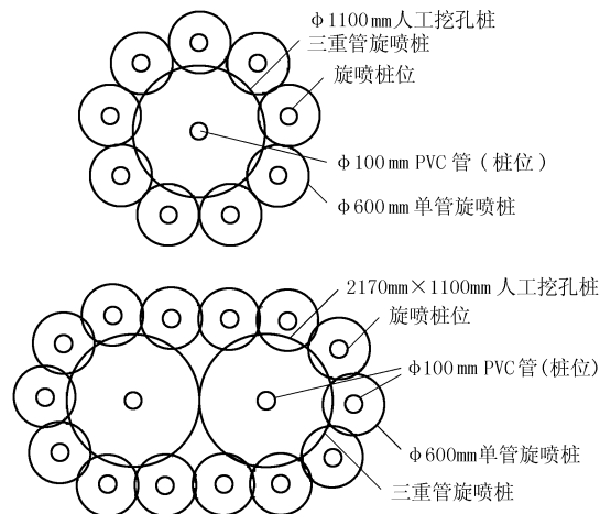
图 1 旋喷桩加固桩位布置示意图
